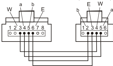
RJ45-Stecker (Vorderansicht)
