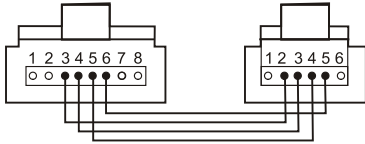
RJ45-Stecker (Vorderansicht)
