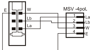
TAE 6F-Stecker (Vorderansicht)
